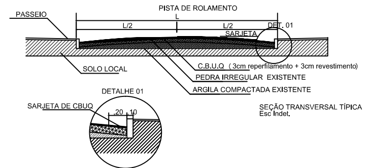
SEÇÃO TRANSVERSAL
