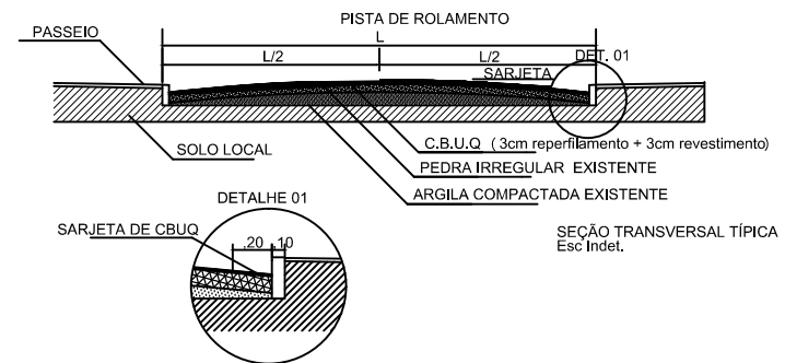
SEÇÃO TRANSVERSAL
