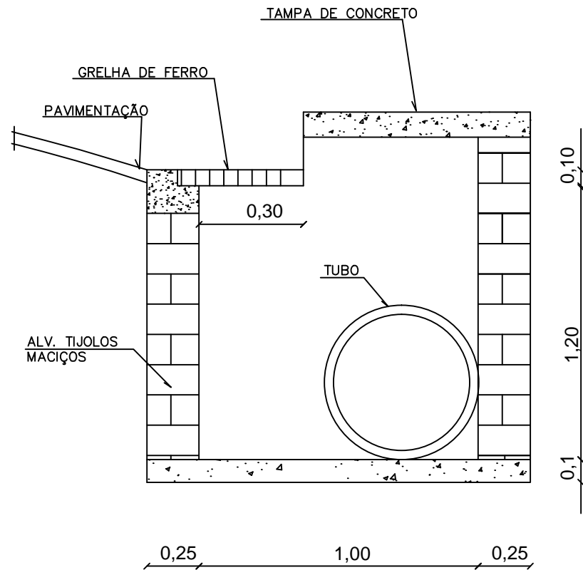
CORTE AB
