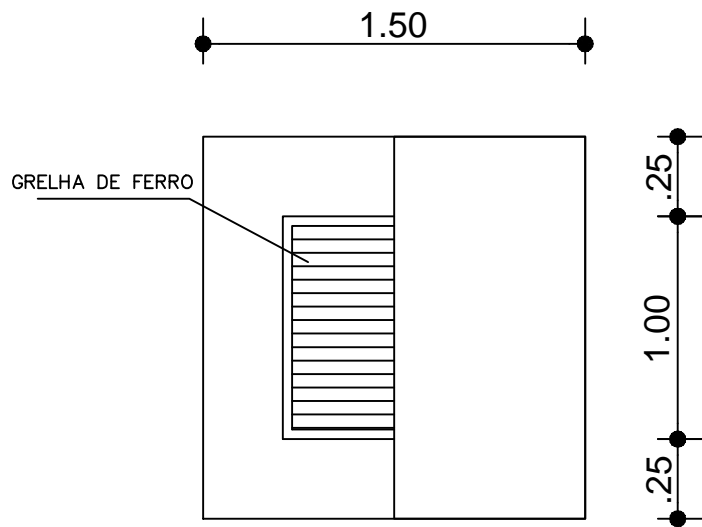
CAIXA DE CAPTAÇÃO PLANTA BAIXA
