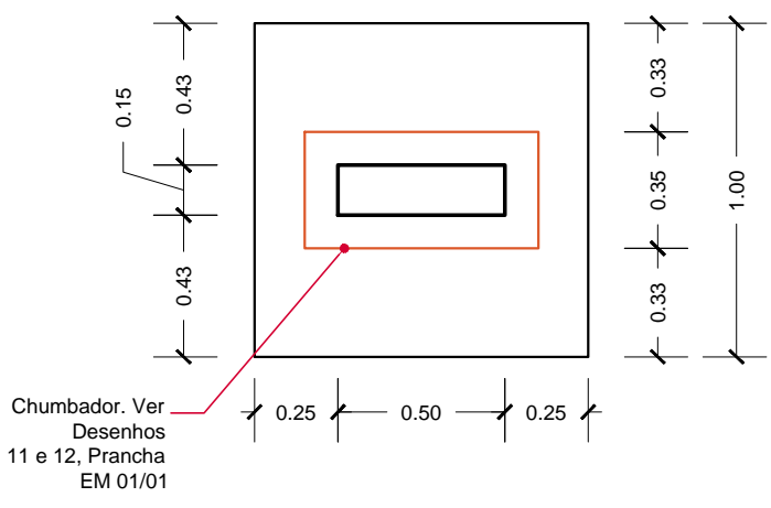
01 BLOCO B01 - 04 Unidades Escala 1:10
