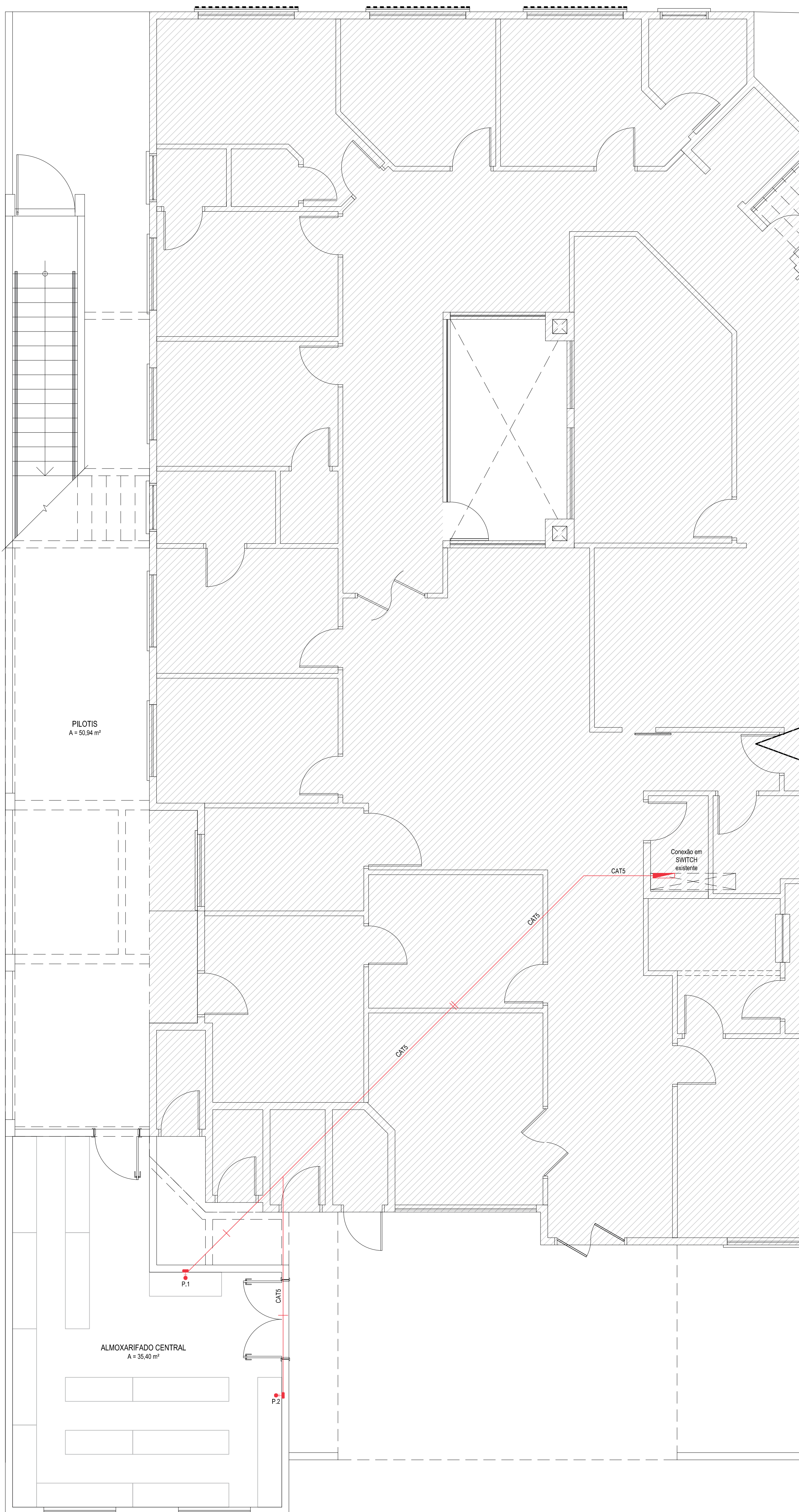
01 PLANTA LÓGICA PAV. TÉRREO ESCALA 1:50
