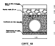
ENCHIMENTO DE VALA DRENAGEM EM RUAS PAVIMENTADAS
