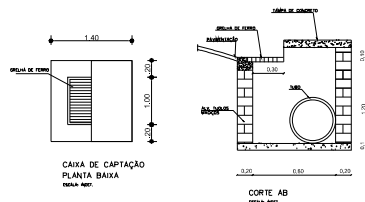
DETALHE DOS DISPOSITIVOS BOCA COLETORA
