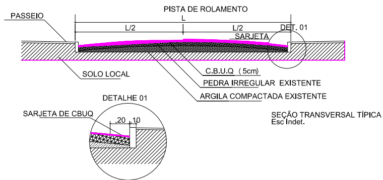
SEÇÃO TRANSVERSAL
